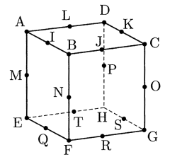
図1: 立方体 ABCD-EFGH
